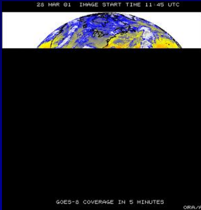
GOES-I/P
